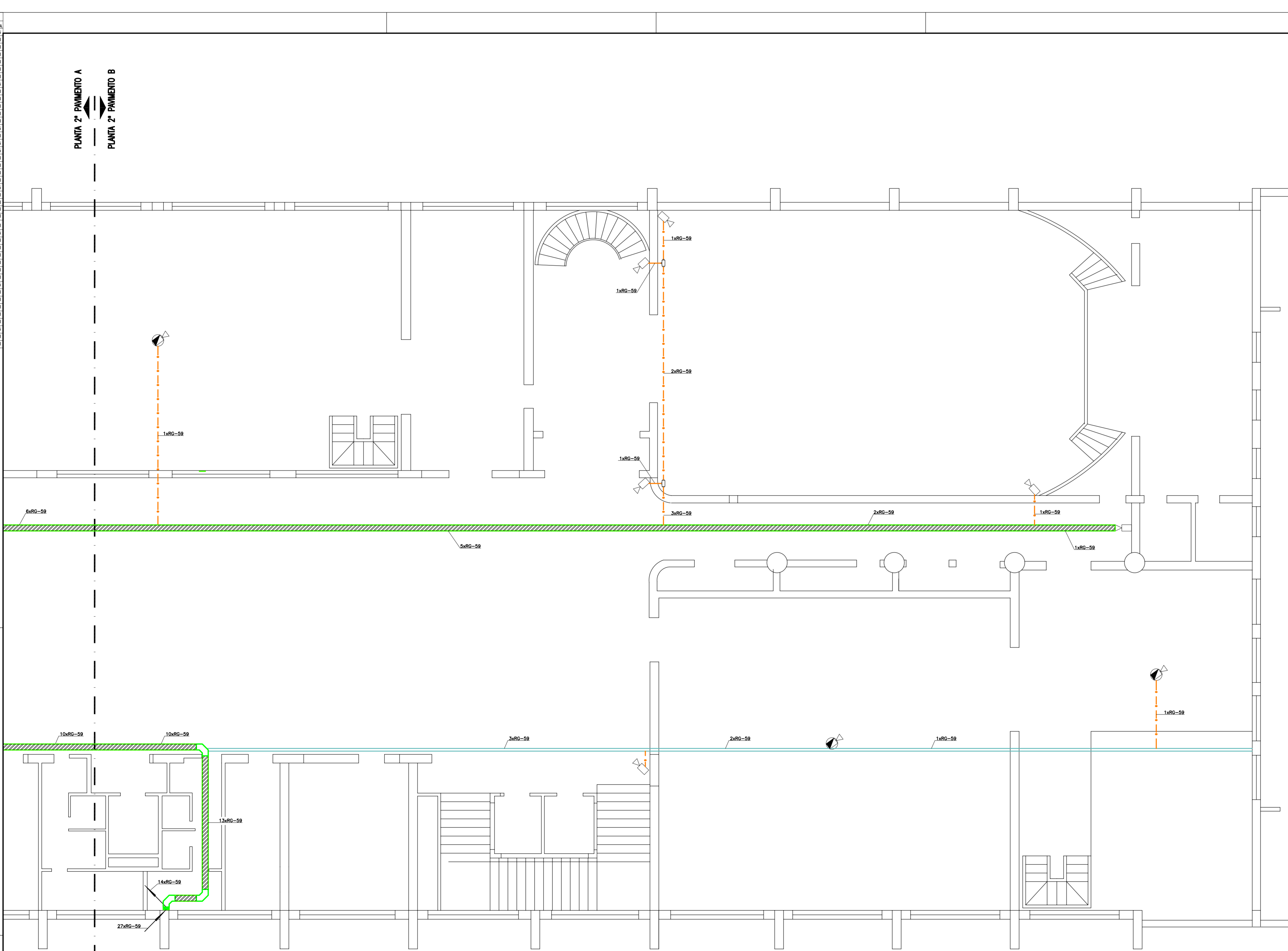
PLANTA 2º PAVIMENTO B ESCALA 1:75
